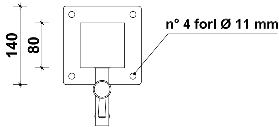
prospetto frontale
