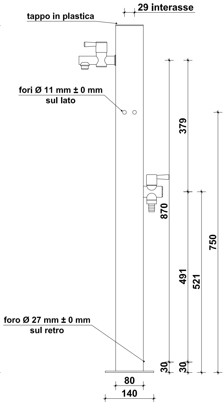
prospetto laterale
